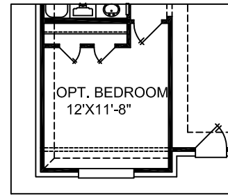
OPTIONAL BEDROOM 5
